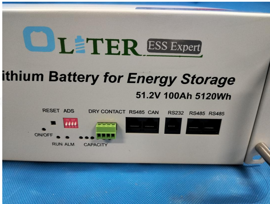
EUT Photo 5
